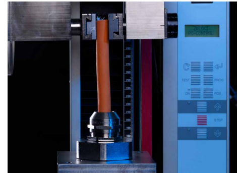
Zugprüfung / Tensile resistance
