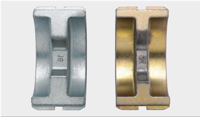
Kuva 6: Alumiini- ja kuparipuristusleuat
