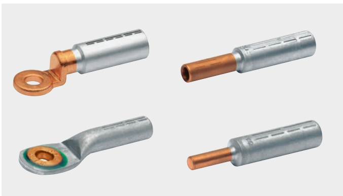
Kuva 1: Al/Cu -kaapelikengät, -vaihtoliitin ja tappiliitin
