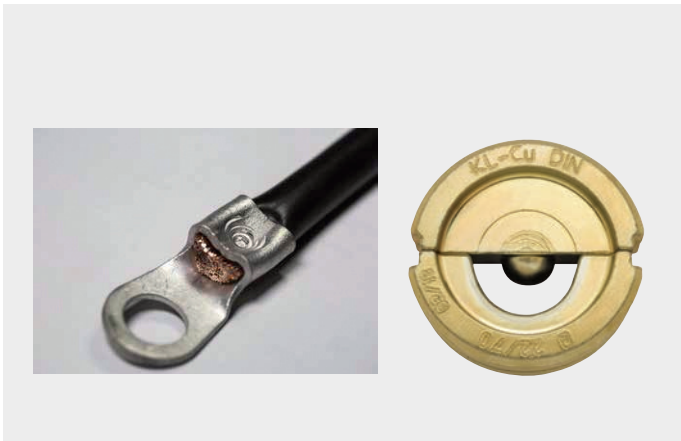
Kuva 12: Tuurnapuristettu levykaapelikengä ja tuurnapuristusleuat
