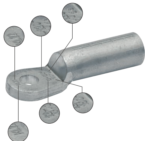
Kuva 5: Alumiinikaapelikengä, merkinnät
